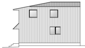
北立面図
